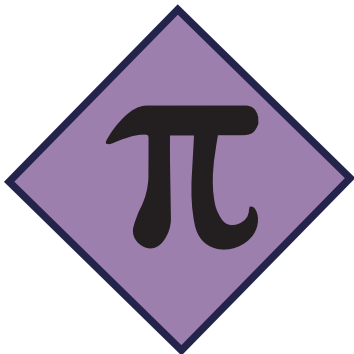
Matemáticas - Física
