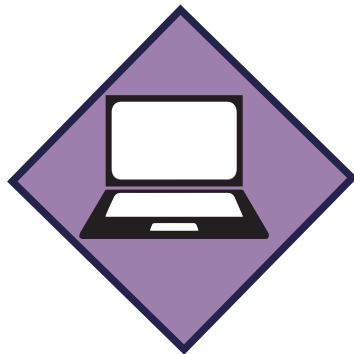
Computación
