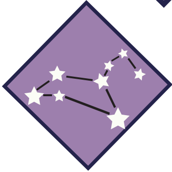
Astronomía
