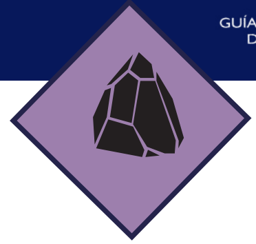
Geología
